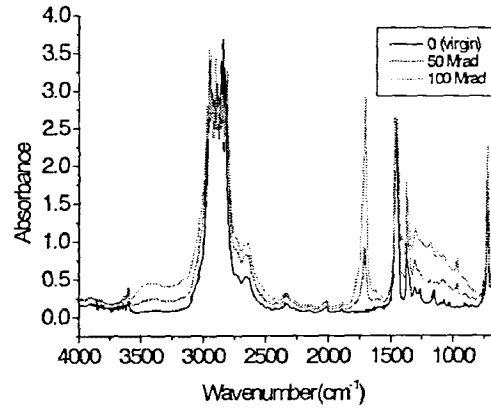
그림 5. 방사선 조사된 XLPE 시료의 IR 스펙트럼 Fig. 5. IR spectrum of \gamma -ray irradiated XLPE
