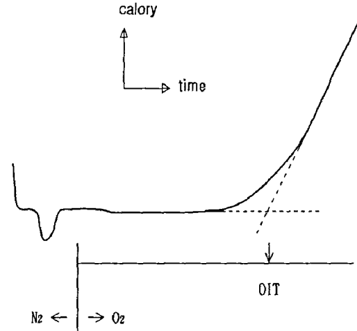
그림 1. 산화유도시간 측정 예
