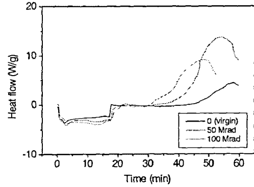
그림 4. 방사선 조사된 EPDM 시료의 DSC thermogram
