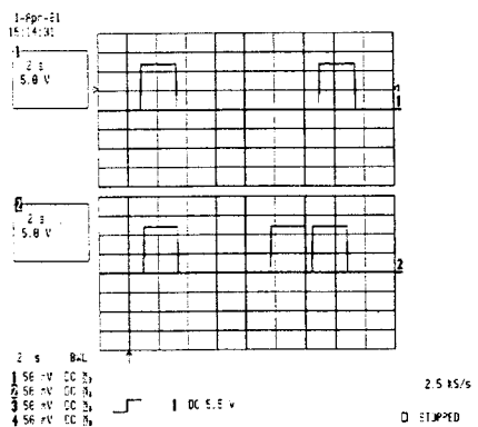
그림 6 The case of shield and not shield when the spread of fire
