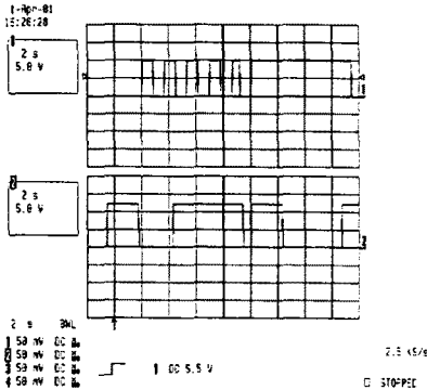
그림 7 UV, IR Output before filtering
