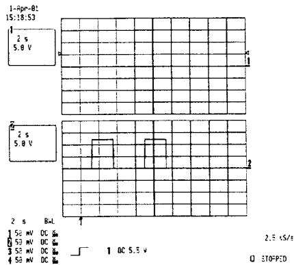
그림 5 The case of shield(a) and not shield(b)
