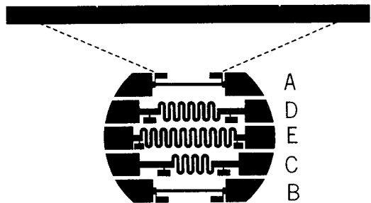
그림 1. 초전도 한류 fuse의 패턴모양
