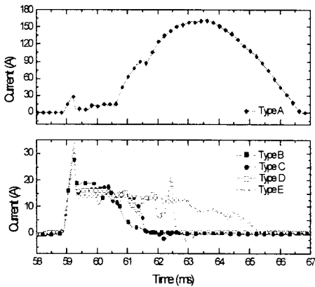
그림 3. 각 초전도 fuse의 한류 및 방전특성
