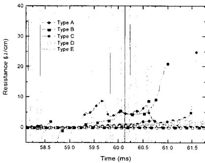
그림 4. 각 초전도 fuse의 단위길이당 저항특성
