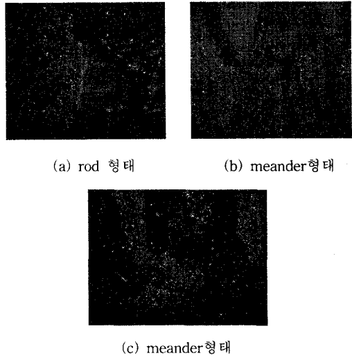
그림 5. 각 초전도 fuse의 용단된 부분의 사진
