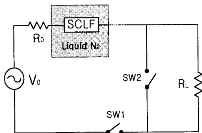
그림 2. 초전도 fuse의 실험 회로도
