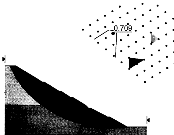
Figure 8. A slow gradient method(1 : 1.5)
