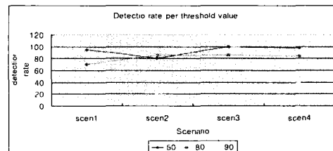
그림6. 임계값 별 침입 탐지율 변화
