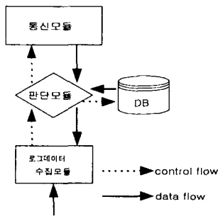
그림2. 에이전트 모듈 내부구조
