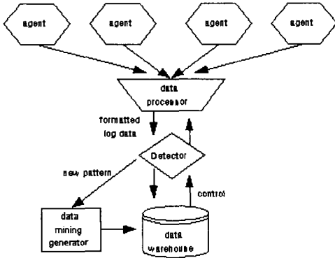
그림3. 제안된 IDS 구조
