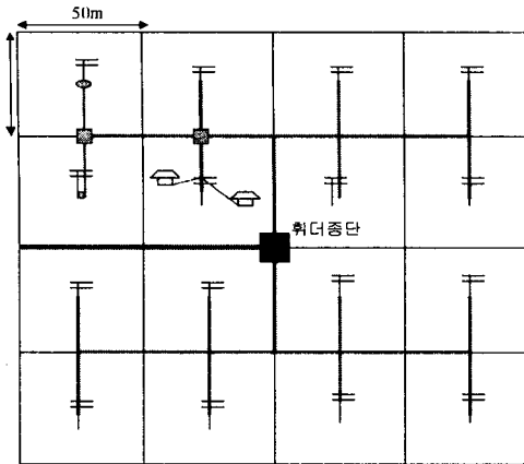
그림 1. 배선망 구성방법
