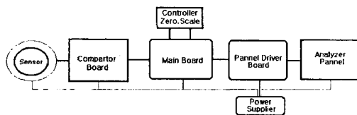
그림 1. TMS 시스템의 하드웨어 구성도
