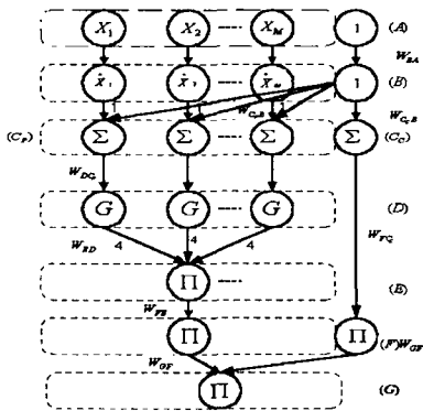
그림 4. Neuro-Fuzzy Model 구성도
