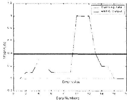
그림 11. 뉴로-퍼지 진단모델의 진단출력 결과
