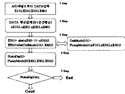
그림 6. Flow-Chart of Diagnosis Algorithms
