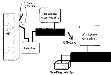
그림 2. 실험장치 구성도
