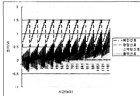
그림 3. 입력신호의 관계
