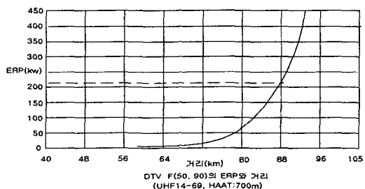
그림 3. DTV F(50, 90) 커버리지와 ERP(CH14~69)
