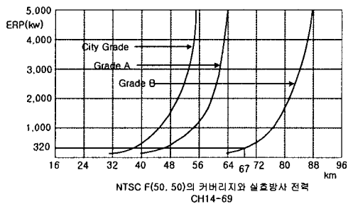
그림 4. NTSC F(50, 50) 커버리지와 ERP
