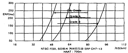
그림 2. NTSC F(50, 50) 커버리지와 ERP(CH2~6)
