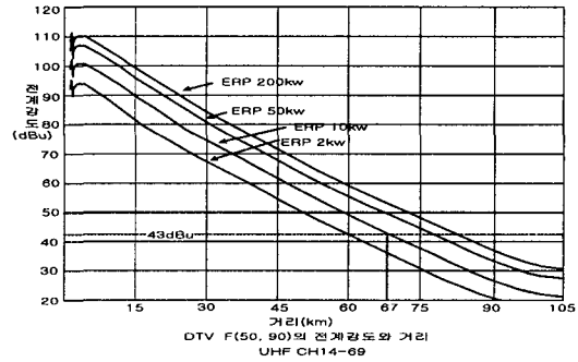
그림 5. DTV F(50, 90) 전계강도와 거리(CH14~69)
