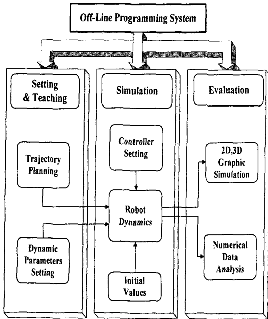
그림 2. 오프라인 프로그래밍 시스템의 구성
