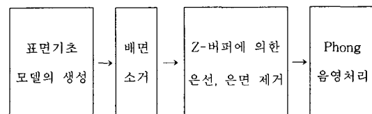
그림. 1 음영처리 흐름도
