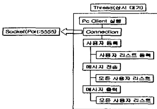
[그림7] PC Client 흐름도
