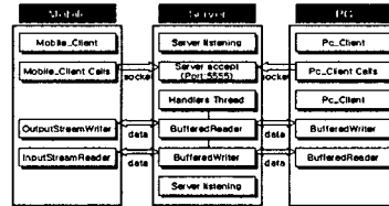
[그림11] 인터넷 통신 과정
