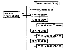
[그림9] Mobile Client 흐름도
