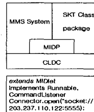
[그림8] Mobile Client 구성도
