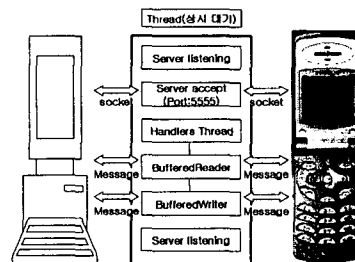
[그림10] Server 흐름도
