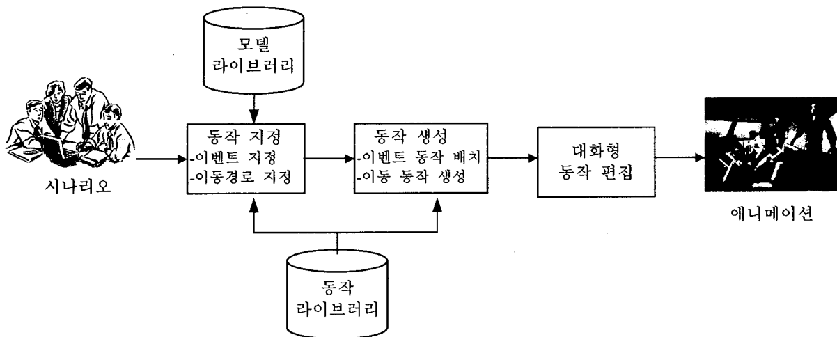
그림 1. 사건 재연 시스템 구성도
