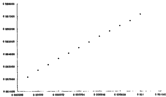
그래프 1 열전대감지기(x축)과 직류전압계(y축)의 관계
