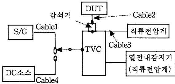
그림1. 시스템의 구성도
