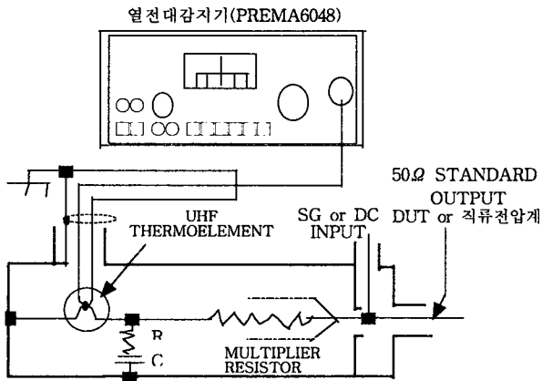
그림2 TVC의 내부구조
