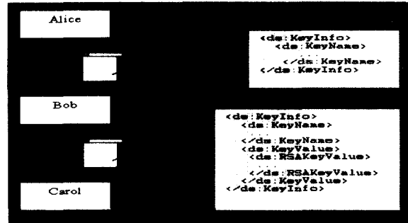
[그림 2] <ds:KeyInfo>내부의 전송 메시지에 대한 예제
