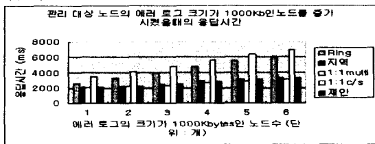
그림5. 관리 대상 노드의 에러 로그 크기가 1000kb인 노드를 증가시켰을 때의 응답시간
