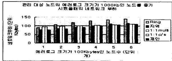
그림6. 관리 대상 노드의 에러 로그 크기가 1000kb인 노드를 증가시켰을 때의 네트워크 부하
