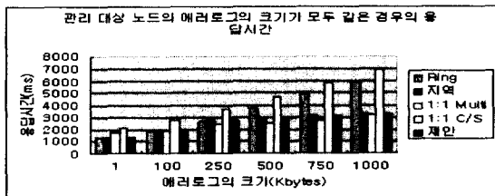
그림4. 관리 대상 노드의 에러 로그 크기가 모두 같은 경우
