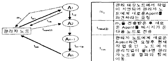
그림 2 관리 대상 노드의 지역 계산 시간에 따른 에이전트 파견방법.
