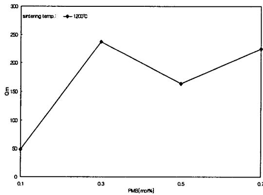
그림 3-3. xPMB-(1-x)PZT계 세라믹의 기계적 품질계수(Qm) (x=0.01, 0.03, 0.05, 0.07 mol%)
