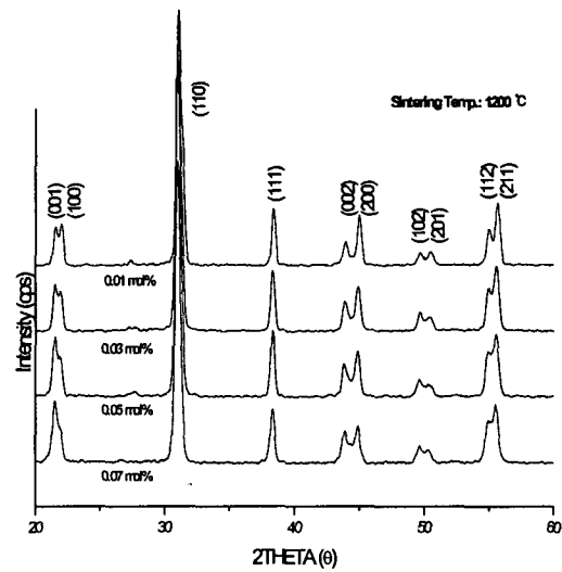
그림 3-1. xPMB-(1-x)PZT계 세라믹의 XRD pattern (x=0.01, 0.03, 0.05, 0.07 mol%)
