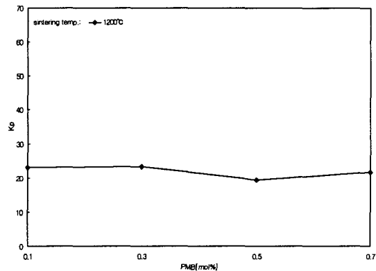
그림 3-2. xPMB-(1-x)PZT계 세라믹의 전기기계 결합계수(kp) (x=0.01, 0.03, 0.05, 0.07 mol%)
