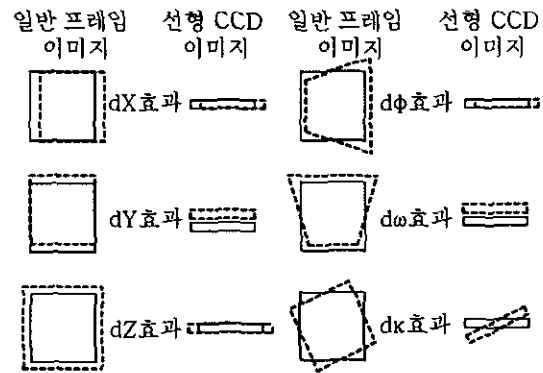
그림 2. 프레임과 선형 CCD 영상에서 외부표정 요소에 의한 효과 1)
