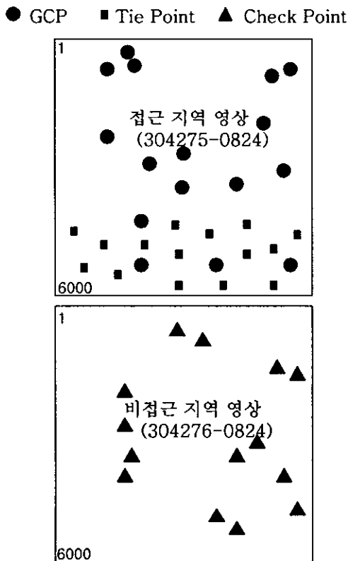
그림 10. GCP, Tie Point 및 Check Point 배열
