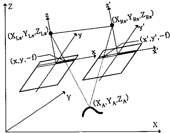
그림 9. 선형 CCD영상 삼각측량
