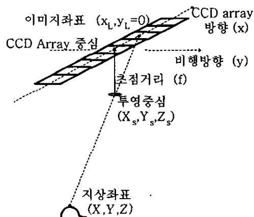
그림 1. Pushbroom 위성영상 공선조건식
