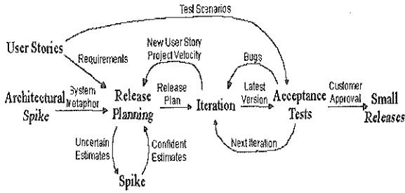
그림 1 Extreme Programming Project
