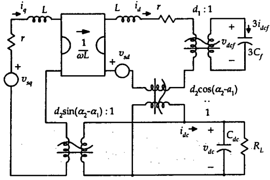
Fig. 4. Circuit DQ transformation.
