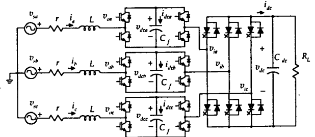
Fig. 1. Hybrid cascade 5-level PWM rectifier.
