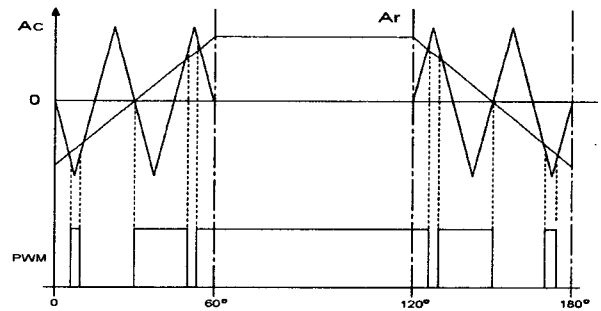
그림 4 PWM방식의 싸이리스터 컨버터 Fig. 4 Trapezoid pwm method
