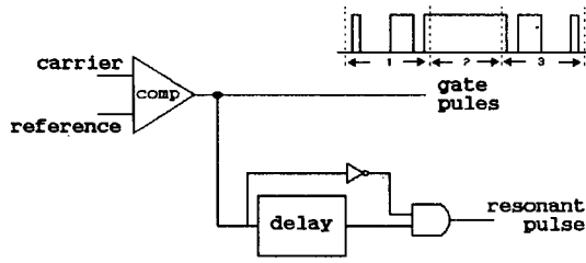
그림 5 PWM 펄스 발생기 Fig. 5 PWM pulse generator
