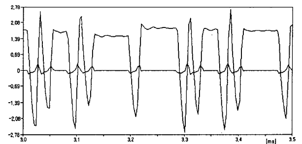
(b) 공진캐피터 전압 전류
