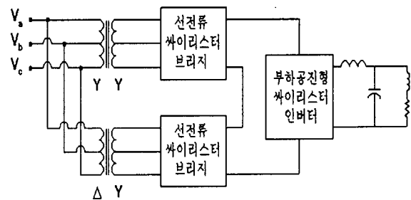
그림 1 저주파 유도가열기 전력변환기 Fig. 1 Low-frequency Induction heating system
