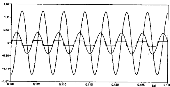
(f) 인버터 출력 전압 전류
