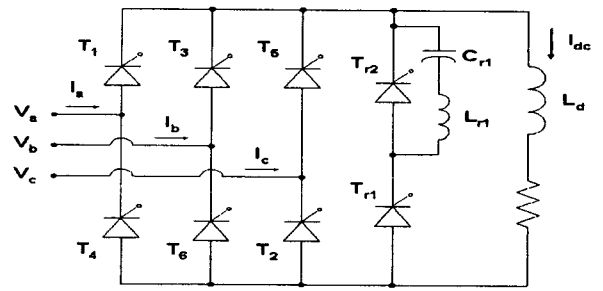
그림 3 싸이리스터 PWM 컨버터 Fig. 3 Thyristor PWM converter
