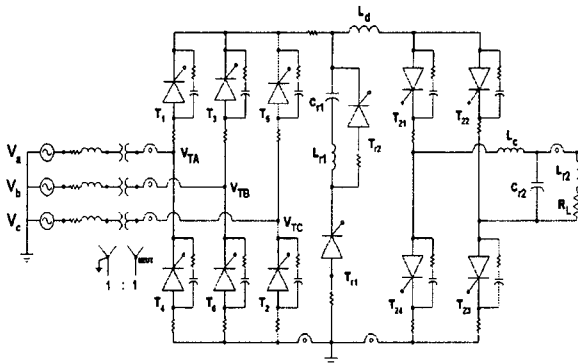
그림 6 시뮬레이션 모형 Fig. 6 Simulation model
