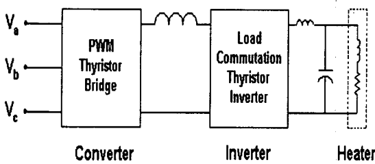
그림 2 제안하는 전력변환기 Fig. 2 Configuration of heating system
