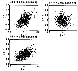
그림 7. 진동신호의 포엔카레 단면
