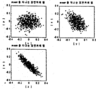
그림 6. 진동 신호의 포엔카레 단면
