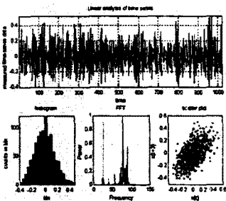
그림 2. 베어링 진동신호의 시계열과 히스토그램 FFT, 재구성한 어트랙터,
