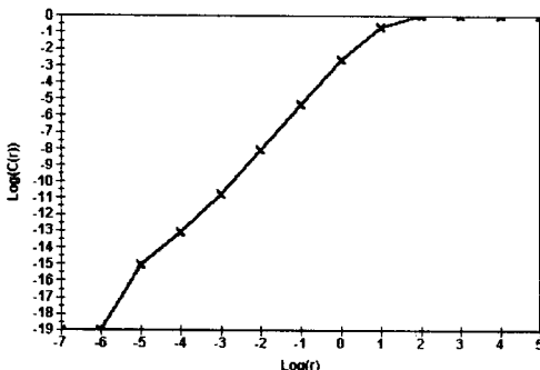
그림 7. 상관 차원
