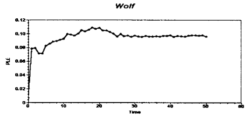
그림 9. 리아프노프 지수
