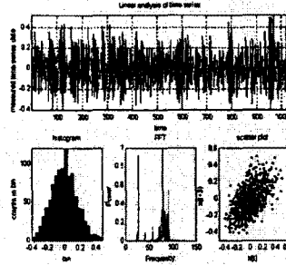
그림 3. 베어링 진동신호의 시계열과 히스토그램, FFT, 재구성한 어트랙터
