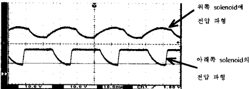
그림 7 36Hz일 때 armature가 위쪽 solenoid에 붙었을 때 상·하 solenoid의 전압 파형
