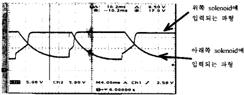
그림 6 35Hz에서 상·하 solenoid의 전압파형
