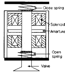
그림 1 EMV 시스템의 구성도
