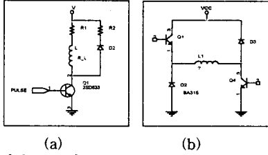
그림 4 기본 구동회로
