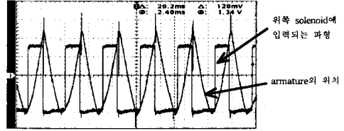
그림 8 상부 solenoid에 입력되는 전압파형과 armature의 위치파형
