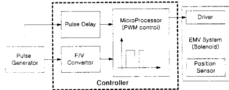
그림 3 EMV 제어 블록도
