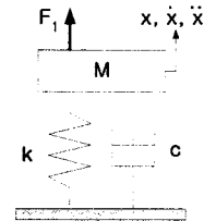
그림 2 EMV 시스템의 모델링
