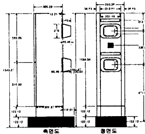
그림. 3 단말기 외면도 Fig. 3 Terminal Output
