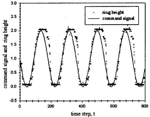
그림 7. 입력신호와 링의 위치
