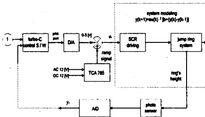
그림 6. 점핑링 시스템 모형화 블록선도
