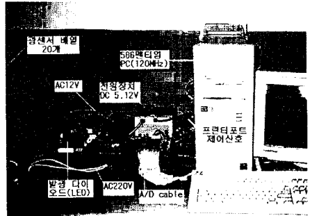
그림 4. 광 센서의 인터페이스 회로와 제어보드 Fig. 4. Photo sensor interface and control board
