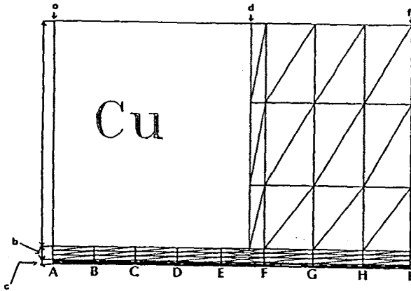
a : Copper knife electrode b : Air gap c : Specimen
