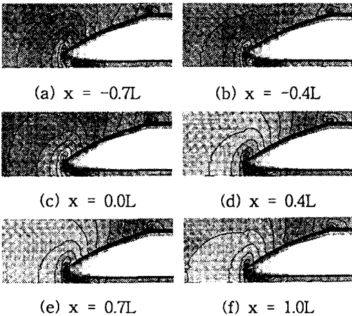
Fig. 10 진입에 따른 전두부 압력분포 변화
