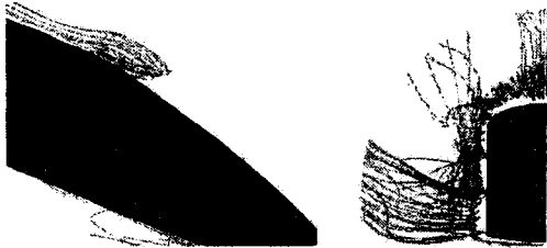
(a) 전두부 경사보기 (b) 전두부 정면보기 Fig. 6 관성좌표계 전두부 유선분포
