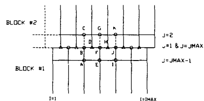
Fig.2 Sliding Multi Block 도식도
