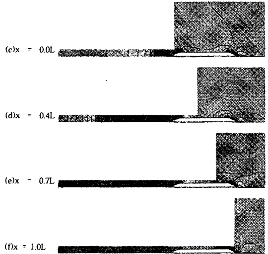
Fig. 8 진입에 따른 대칭면 압력분포 변화
