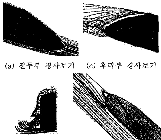
(b) 전두부 정면보기 (d) 후미부 상면보기
