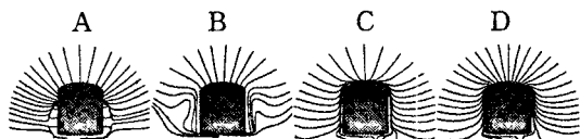
Fig. 7(a) x = -0.7L 에서의 횡단면 유선분포
