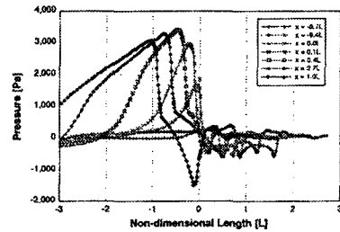
Fig. 9 진입에 따른 내부 압력변화
