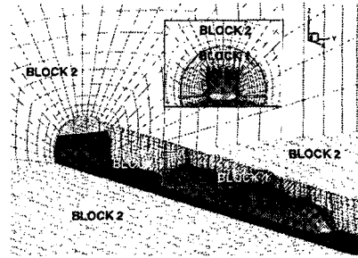
Fig.1 고속전철과 터널의 격자계
