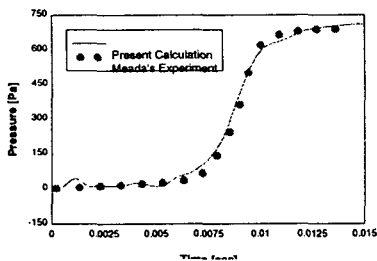
Fig.3 터널내부 압력 변화의 비교
