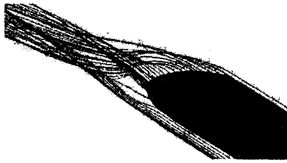
(e) 후미부 후류영역 경사보기 Fig. 5 전철주위 유선분포
