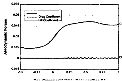
Fig.12 진입에 따른 공기역학적 힘의 변화
