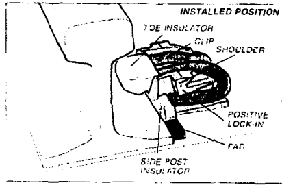
그림 3 Pandrol Fastclip
