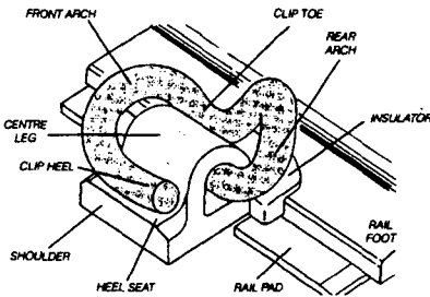
그림 1 Pandrol type PR series clip
