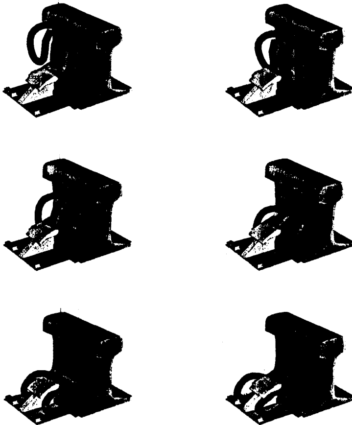
그림 7. 레일체결장치 역방향 체결방식의 설머
