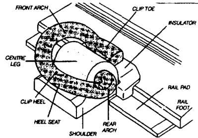
그림 2 Pandrol type 'e' series clip
