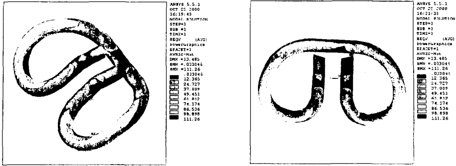
그림 9. Simple beam의 응력도
