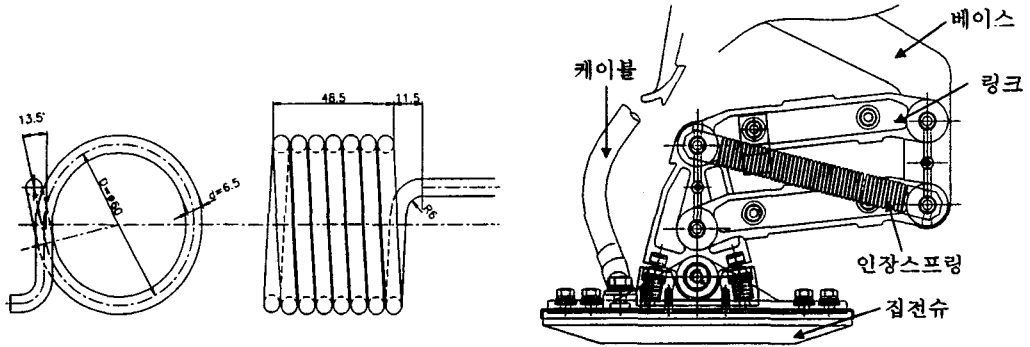
(a) 측면상방향 집전장치의 비틀림스프링 (b) 횡방향 집전장치의 인장스프링 그림 7 접촉력 유지를 위한 스프링
