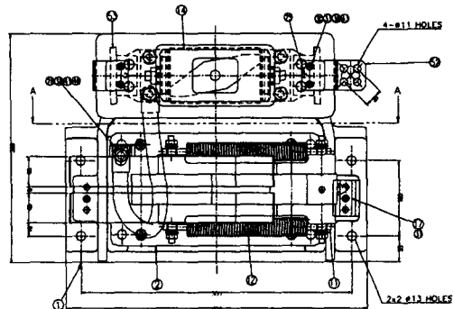
(b) 횡방향 집전장치
