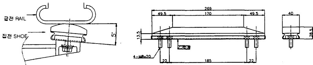
(a) 측면상방향 집전장치
