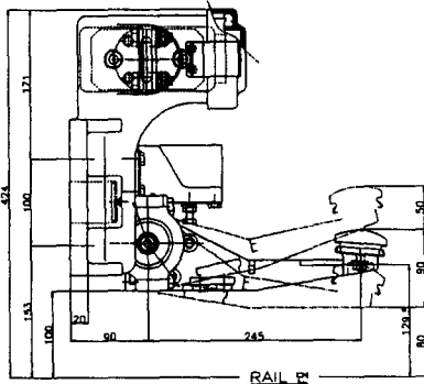
(a) 측면상방향 집전장치
