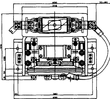
(a) 측면상방향 집전장치
