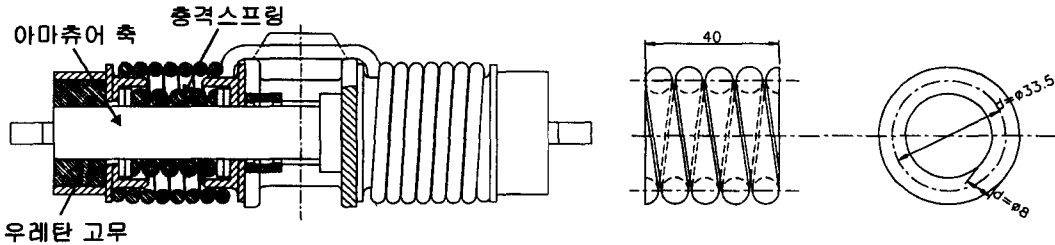
(a) 진동 및 충격흡수를 위한 축설계
