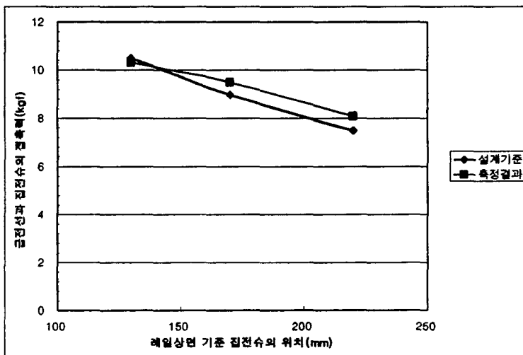
그림 10 측면상방향 집전장치의 접촉력 변화
