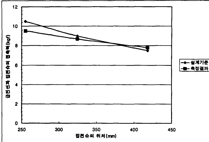
그림 11 횡방향 집전장치의 접촉력 변화
