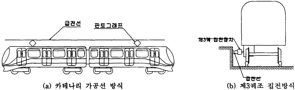
그림 1 도시철도의 집전방식 유형
