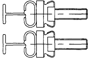
그림 5 횡방향 집전장치와 급전선의 접촉
