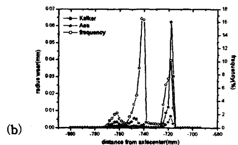
그림. 13 (a) 1,200km 주행시 프로파일 (b)기존선 주행시 왼쪽차륜 마멸량 및 접촉빈도분포
