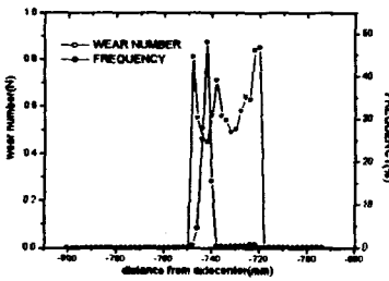
그림.10 고속선 주행시 왼쪽차륜 마멸지수 및 접촉빈도분포
