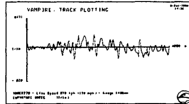
그림. 3 고속선 선로 곡률변화
