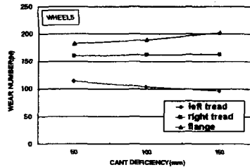
그림. 16 해석구간 캔트량변화 그림. 17 캔트부족량에 따른 5번차륜 마멸수 변화
