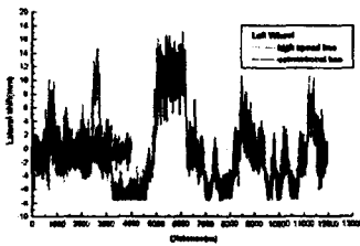
그림. 4 왼쪽차륜 횡변위
