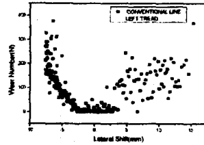
그림. 9 기존선 주행시 왼쪽차륜 마멸지수 분포
