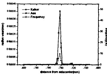
그림. 12 (a) 120,000km 주행시 프로파일 (b)고속선 주행시 왼쪽차륜 마멸량 및 접촉빈도분포
