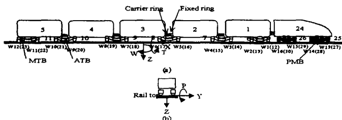
그림. 1 차량모델 : 동력차+동력객차+객차+객차+객차+동력객차
