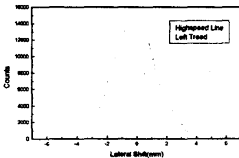
그림. 6 고속선 주행시 왼쪽차륜 횡변위 분포
