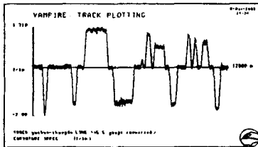
그림. 2 유천-청도구간 곡률 변화
