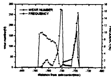
그림. 11 기존선 주행시 왼쪽차륜 마멸지수 및 접촉빈도분포
