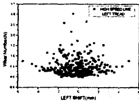
그림. 8 고속선주행시 왼쪽차륜 마멸지수 분포
