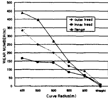
그림. 14 곡선반경에 따른 5번차륜 마멸수 그림. 15 곡선부 유효시와 비유효시 5번차륜 마멸수
