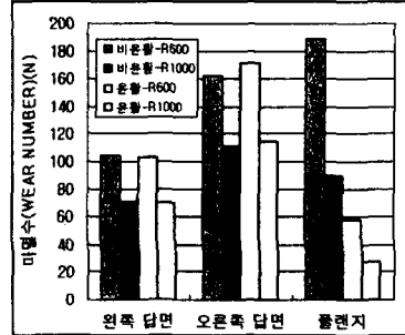
그림. 14 곡선반경에 따른 5번차륜 마멸수 그림. 15 곡선부 유효시와 비유효시 5번차륜 마멸수
