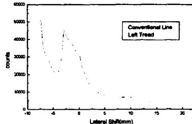
그림. 7 기존선 주행시 왼쪽차륜 횡변위 분포
