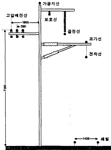
그림 1. 전차선로의 수직배치도
