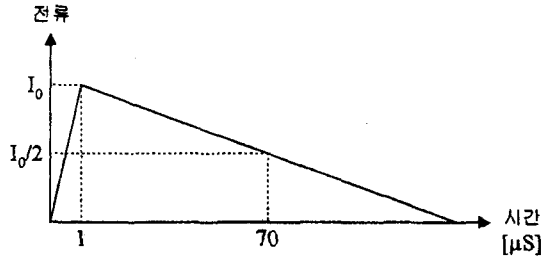
그림 3. 뇌격전류파형
