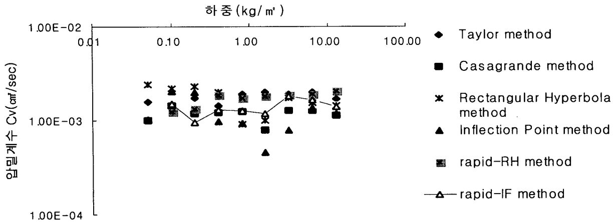
그림 6. 울산B 시료의 시험방법에 따른 압밀계수 ( C_v )의 변화
