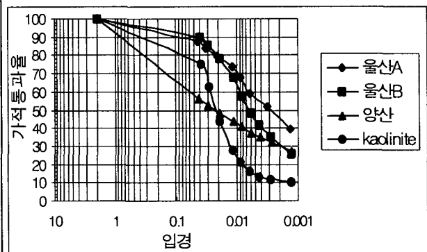
그림 5. 입도분포곡선
