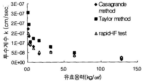
그림 9. 울산B시료의 투수계수 변화
