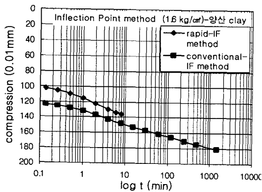
그림 3. 압축량-시간 그래프(양산시료)
