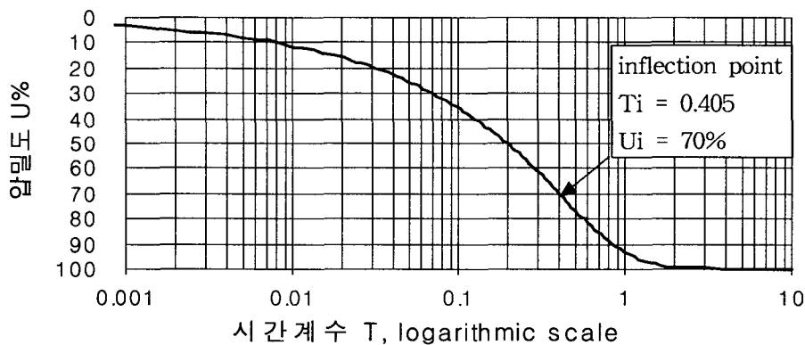
그림 1. 이론적인 압밀 곡선
