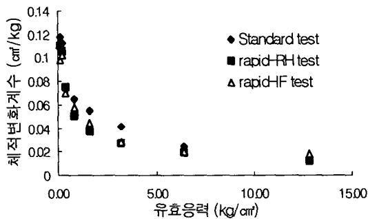
그림 8. 울산B시료의 체적변화계수 변화
