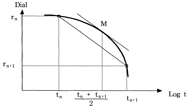
그림 2. 압축-시간곡선에서 기울기 결정
