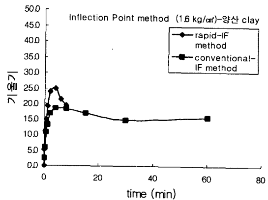
그림 4. 기울기-시간 그래프(양산시료)
