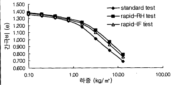
그림 7. 간극비 - 유효응력 (양산시료)
