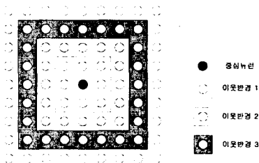
그림 2.2 2차원 배열된 뉴런의 feature map
