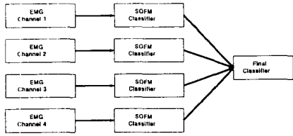
그림 3.1 제안한 EMG 신호분류 방식
