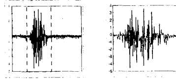
그림 4.1 측정된 EMG 신호 및 주변데이터 제거 후 신호과형
