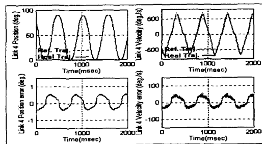
Fig. 10. 무부하 상태에서의 위치와 속도추종에 대한 SOFC의 실험결과
