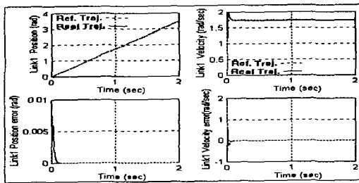
Fig. 7. 램프입력에 대한 4 kg 부하가 있을 때 1축의 위치 및 속도 궤적추종의 시뮬레이션 결과
