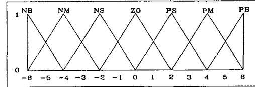
Fig. 3. 언어 변수
