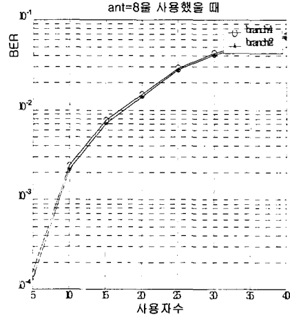
그림 5. 사용자수에 따른 BER
