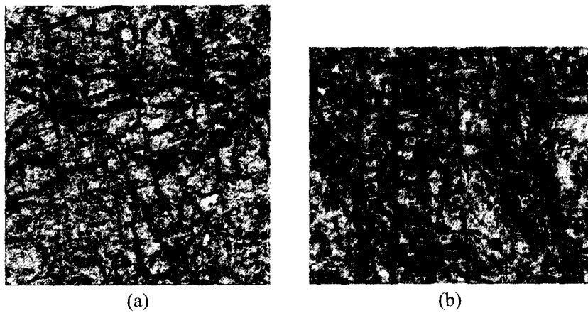
Fig. 14. Sobel edge detector outputs.
