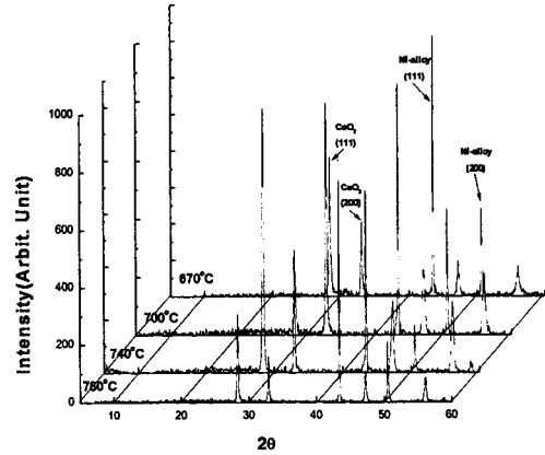
그림 1. 670-780°C에서 증착한 CeO 2 의 XRD 결과
