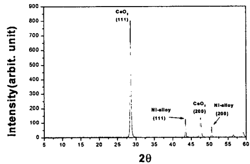
그림 2. 진공상태에서 증착한 CeO 2 의 XRD 결과.
