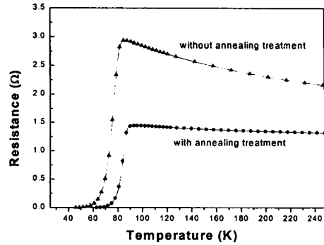
그림 4. 후열처리의 유무에 의한 임계온도의 변화
