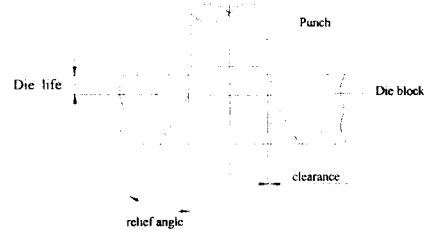
Fig. 3 Clearance, relief angle and die life
