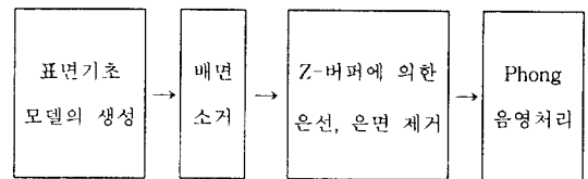
그림. 1 음영처리 흐름도
