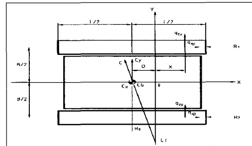
그림 1. 차량선회시 힘의 작용.
