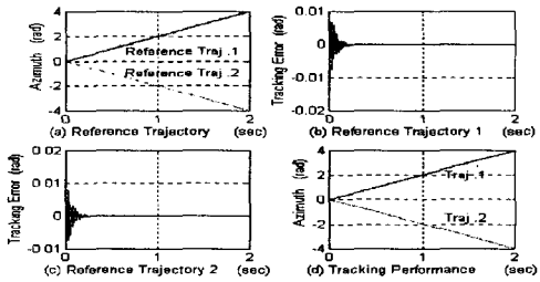
그림 8. 15%의 파라미터의 불확실성을 고려한 NF제어기의 방향각계적추종 제어성능
