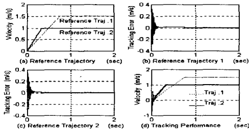
그림 6. 10%의 파라미터의 불확실성을 고려한 NF제어기의 속도계적추종 제어성능
