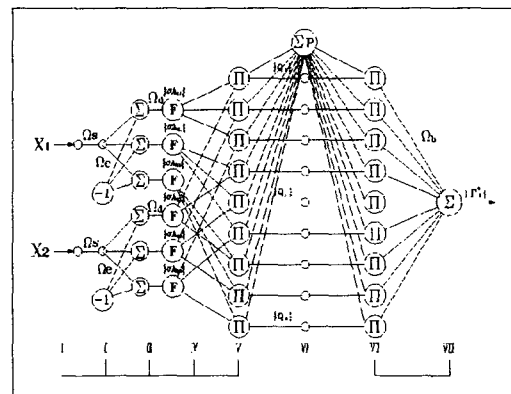
그림 5. 뉴럴-퍼지 네트워크의 기본구조
