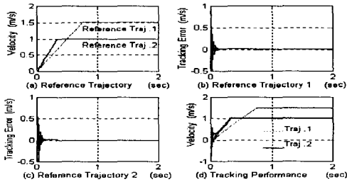
그림 7. 20%의 파라미터의 불확실성을 고려한 NF제어기의 속도계적추종 제어성능
