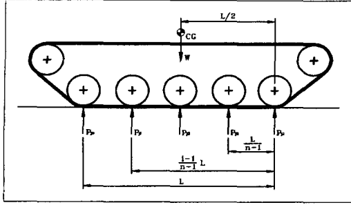
그림 2. 정지상태의 하중분포
