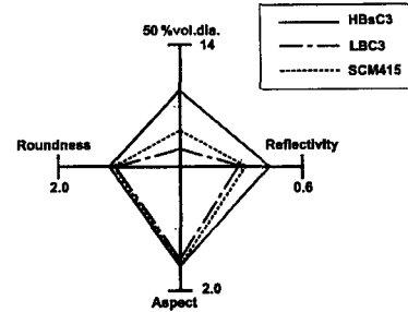
Fig. 8 Diagram of shape parameter
