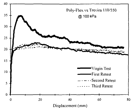
그림 5. 지오멤브레인의 재사용으로 인한 영향 : Poly-Flex 지오멤브레인 vs Trevira 011/550
