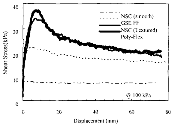
그림 4. 전단응력-수평변위 관계 : 4가지 지오멤브레인 vs Amoco #4510 지오텍스타일
