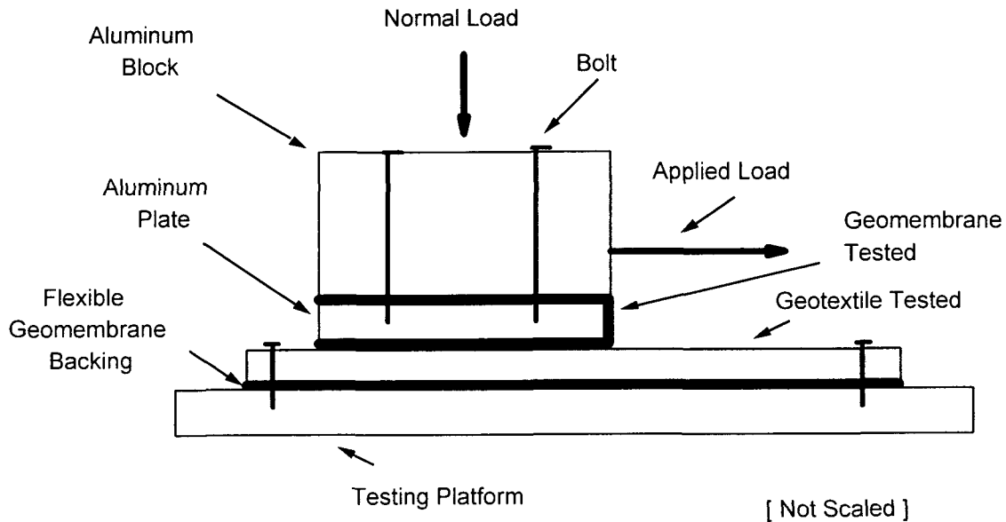
그림 3. 지오멤브레인과 지오텍스타일의 직접 전단 시험기
