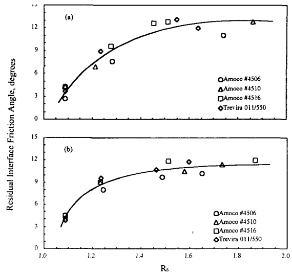
그림 7. 잔류 접촉마찰각과 표면 거칠기와의 관계 (a) 50 Kpa, (b) 100 kPa normal stress
