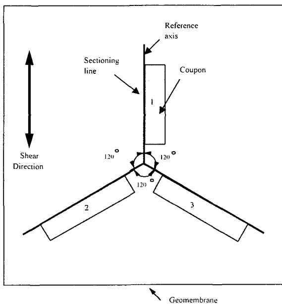
그림 1. 지오멤브레인 시편 선택 방법
