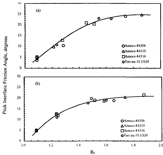
그림 6. 최대 접촉마찰각과 표면 거칠기와의 관계 (a) 50 Kpa, (b) 100 kPa normal stress
