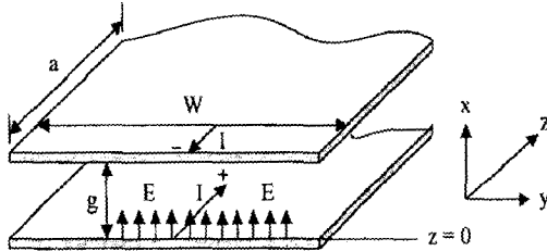
그림 1 평행판 전송선로
