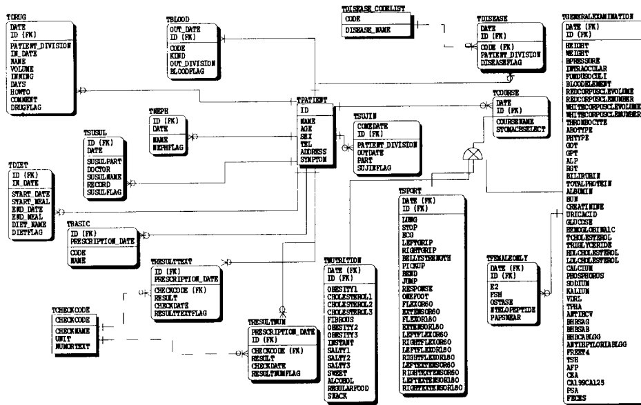
<그림 7> 운영 데이터 창고 스키마
