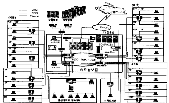
<그림 4> J 병원 시스템 구성도
