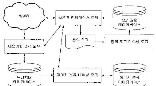
그림 1 데이터마이닝을 이용한 지능적 이미지 검색 시스템
