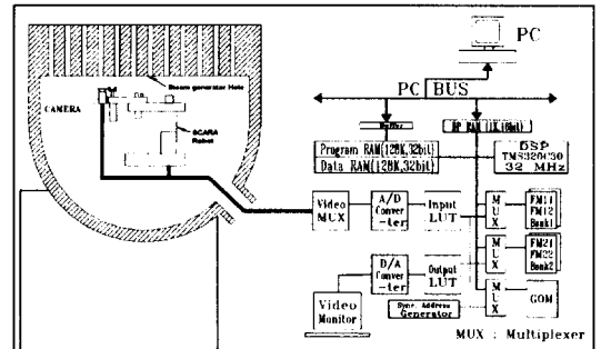
그림. 4. 원자력 발전소의 스텝체너레이터에 대한 비전 시스템의 구조
