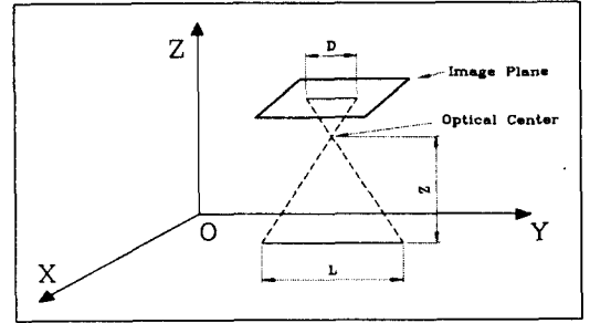
그림. 2. 2, 3차원 라인 및 그 영상구조
