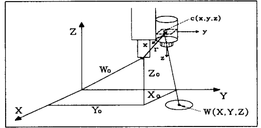
그림. 1. 공간 좌표계 및 카메라 좌표계의 영상기하학
