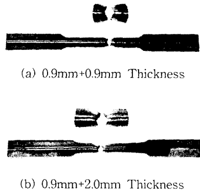
Fig. 6 Fractured specimens by fatigue test Fig. 7은 하중방향과 평행하게 시험편의 길이
