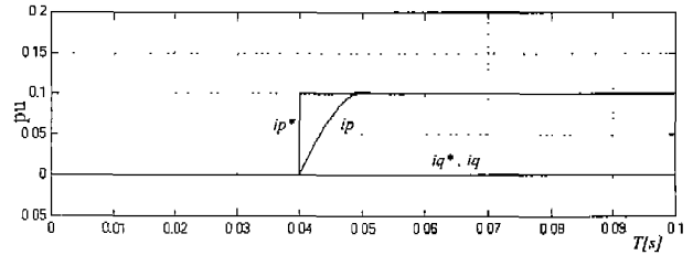
(a) i_p^* 의 스텝응답
