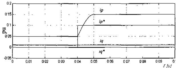
(a) i_p^* 의 스텝응답
