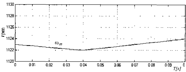
(b) 속도응답
