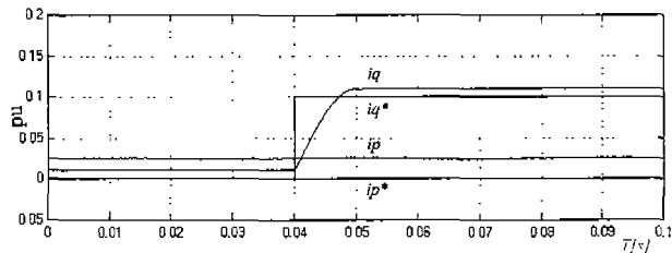
(b) i_q^* 의 스텝응답
