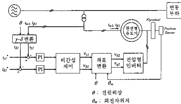
그림 2. 시스템 구성도
