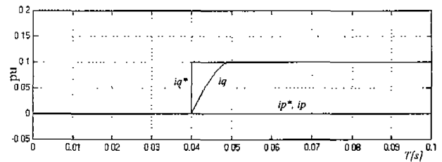
(b) i_q^* 의 스텝응답
