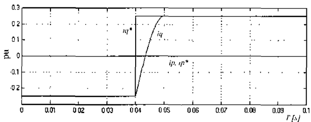
(c) i_q^* 의 스텝응답
