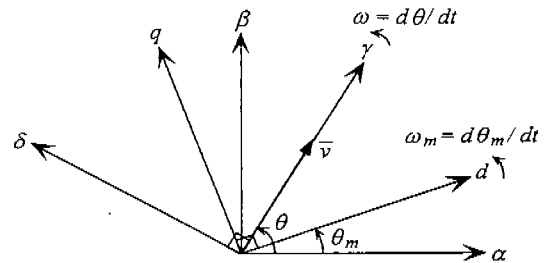
그림 1. 정지좌표계와 회전좌표계
