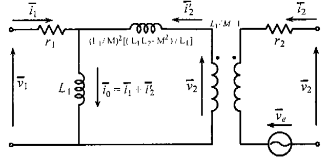
그림 5. 권선형 유도전동기의 등가회로
