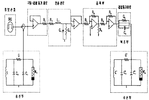
그림7. 등가 전송선로를 가진 비밀통신 회로 Fig.7 Secure communication circuit with equivalent transmission line.
