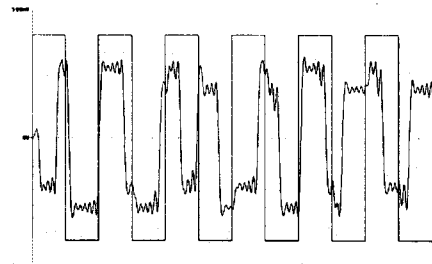
그림 9. 선로 중간에서 도청한 신호 Fig. 9. Wiretapping signal
