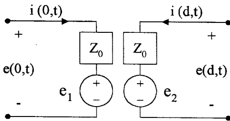
그림 5. 전송 선로의 특성 모델 Fig. 5. The characteristic model of a transmission line
