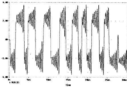
그림 7. 반송파 신호(송신부 신호) Fig. 7. Carrier signal (transmitter signal)
