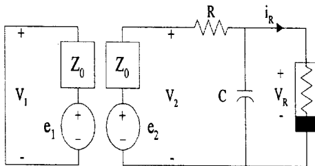
그림 6. 전송 선로를 가진 Chua 회로의 등가회로 Fig. 6. Equivalent circuit of Chua's circuit with a transmission line
