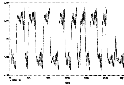
그림 8. 수신부의 카오스 신호 Fig. 8. Chaos signal of receiver signal
