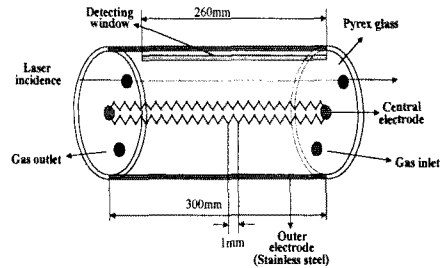
그림 4 방전리액터의 구성도 Fig. 4 Schematic diagram of discharge reactor
