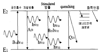
그림 1. 레이저유도 형광(LIF)의 기본원리 Fig. 1 Basic principle of LIF
