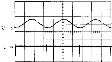
(b) 4 [mA/div], 10[kV/div], 5(ms/div) 인가전압: 3.8 [kV]
