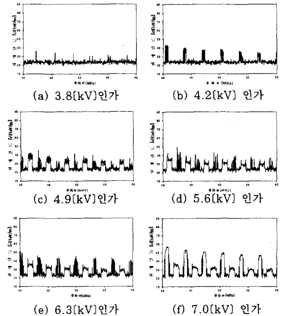
그림 3. 방사전자파 주파수 스펙트럼 분포
