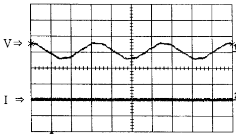
(a) 4 [mA/div], 10[kV/div], 5(ms/div) 인가전압: 3.5 [kV]
