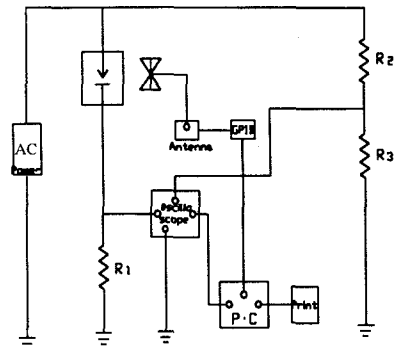
그림 1. 실험회로도
