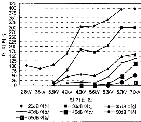
그림 4. 부분방전시 인가전압에 따른 임의의 전계 강도 이상의 데이터 수
