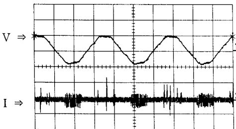
(c) 2 [mA/div], 10[kV/div], 5(ms/div) 인가전압: 6.3 [kV]
