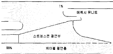
〈그림3〉 등 전위선도 표시
