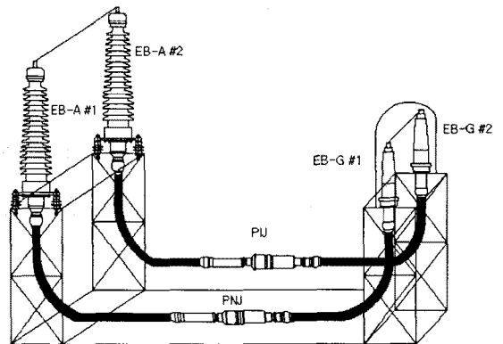
〈그림5〉 조립시험
