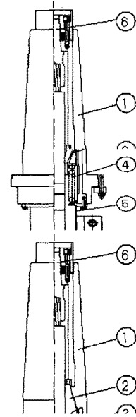
〈그림4〉 66kV SF 6 gas중 종단접속함 (EB-G)
